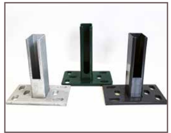
16 Montagefuß für Pfosten 60x40 mm (150x100x8 mm), verzinkt/verz. grün/verz. anthrazit
