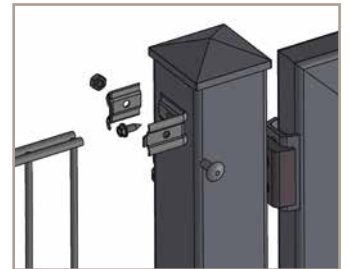
Zaunanschluss
